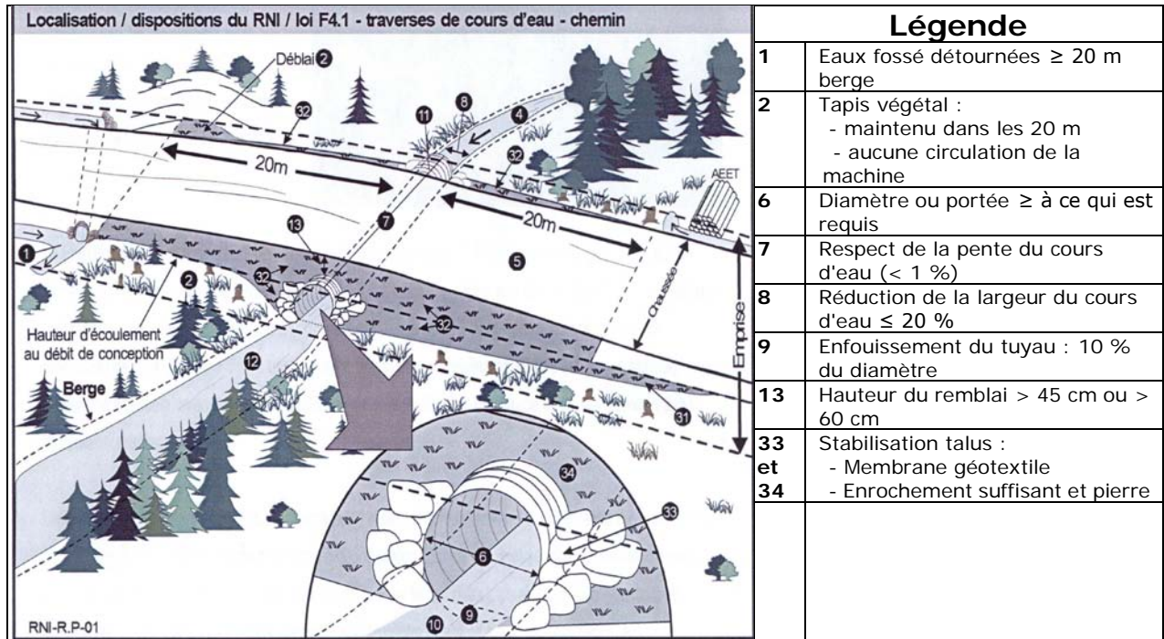
Figure 1 : Exemple d'aménagement d'une traverse de cours d'eau avec un ponceau
